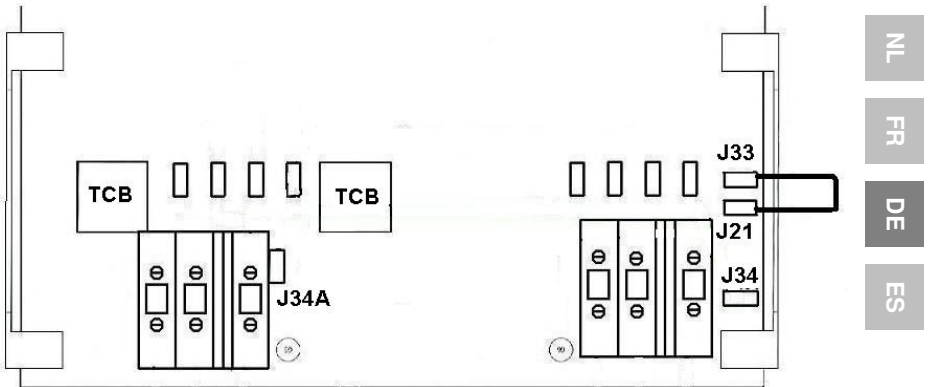
Abb. 5: Fehlerstromschutzschaltung (FI-Schalter)
